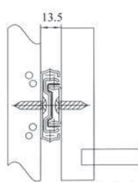
odsazení zásuvky od korpusu (korpus, zásuvka)
